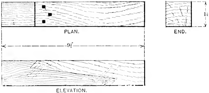
Fig. 187 Scale, 3"=1'
