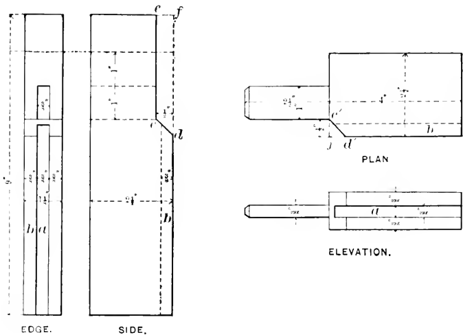
FIG. 216 Scale, 3"=1'
