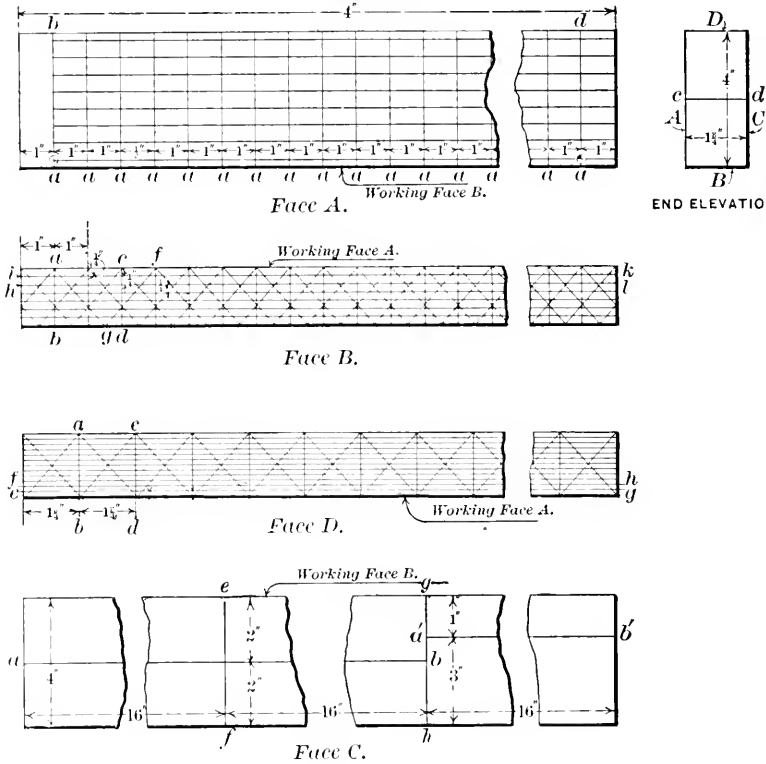
Fig. 137 Scale, 2"=1'
