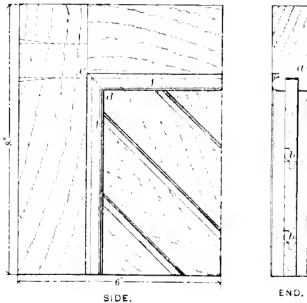
Fig. 215 Scale, 3" 1'
