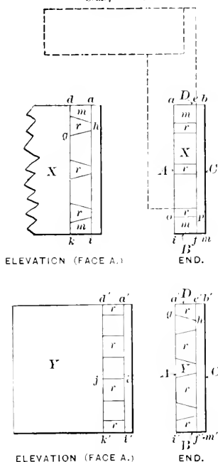
Fig. 206 Scale, 3"=1'
