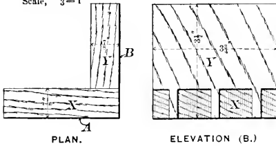
Fig. 199 Scale, 3=1'
