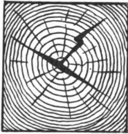
FIG. 42.—Heartshake.
