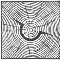
FIG. 45.—Cupshake.
