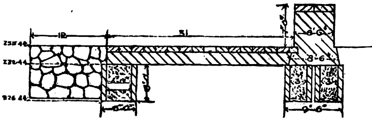
Fig. 23. Coleroon Anicut.
