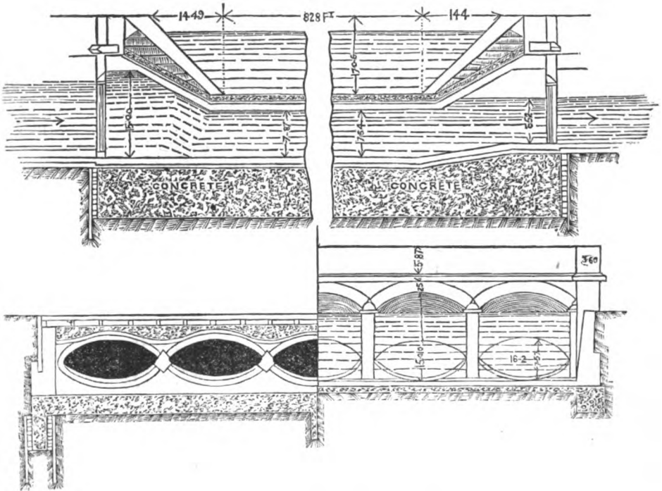
Fig. 79. Sesia Syphon, Cavour Canal.
