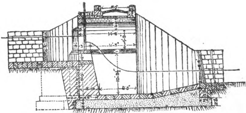
Fig. 62. Canal Fall, Madras.
