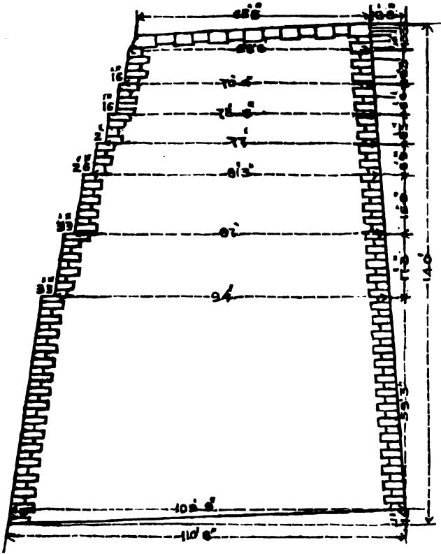
Fig. 126. The Alicante Dam.
