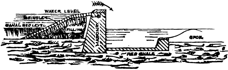
Fig. 20. Jutoor Weir.
