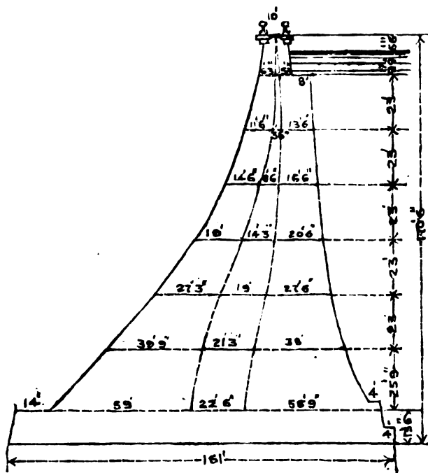
Fig. 123. The Furens Dam.
