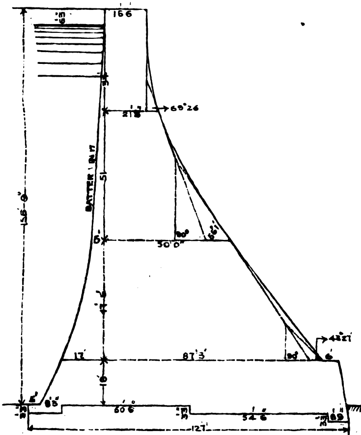
Fig. 124. The Ban Dam.
