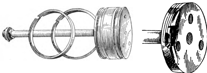
FIG. 48.—Piston.
