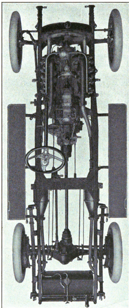
FIG. 118.—Automobile chassis.
