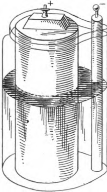
FIG. 233.—Leclanche cell.
