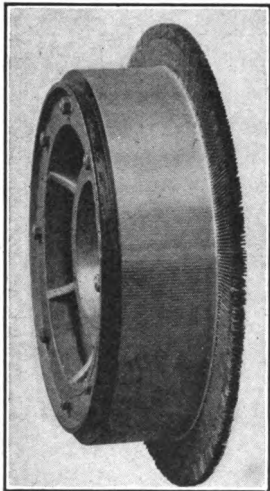
FIG. 243.—Commutator.
