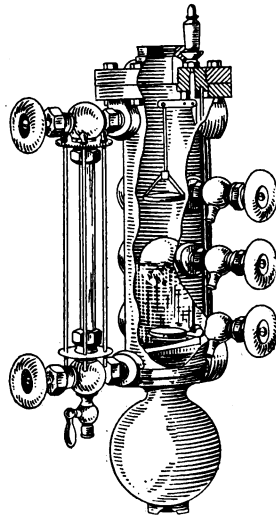
FIG. 27.—Water column.
