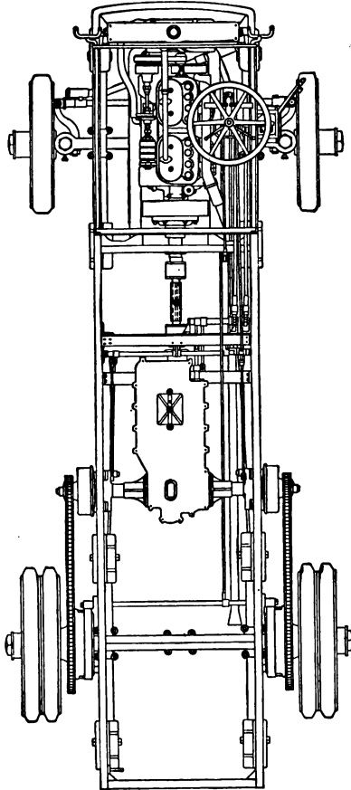
Fig. 119.—Auto-truck chassis.
