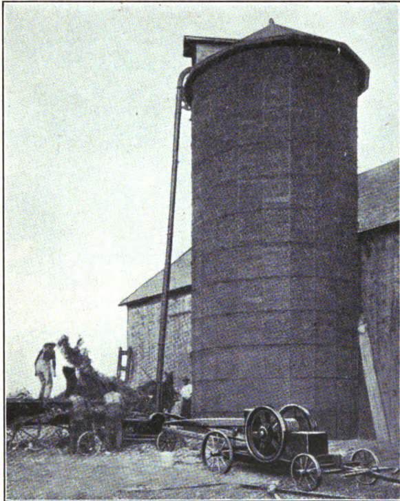
FIG. 110.—Silo filling.
