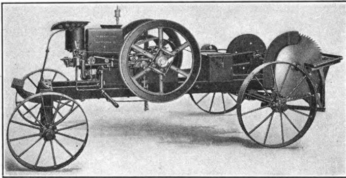
FIG. 117.—Wood-sawing rig.
