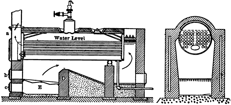
FIG. 4.—Return tubular boiler.
