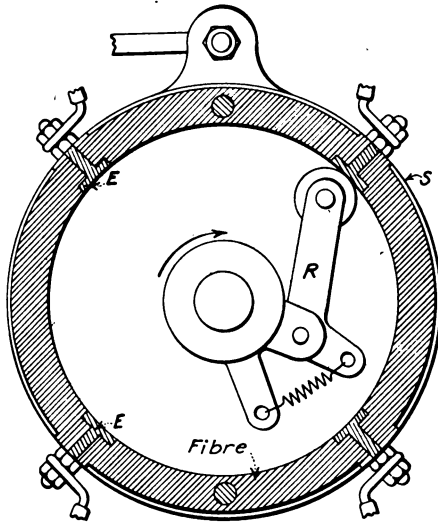
FIG. 102.—Timer.
