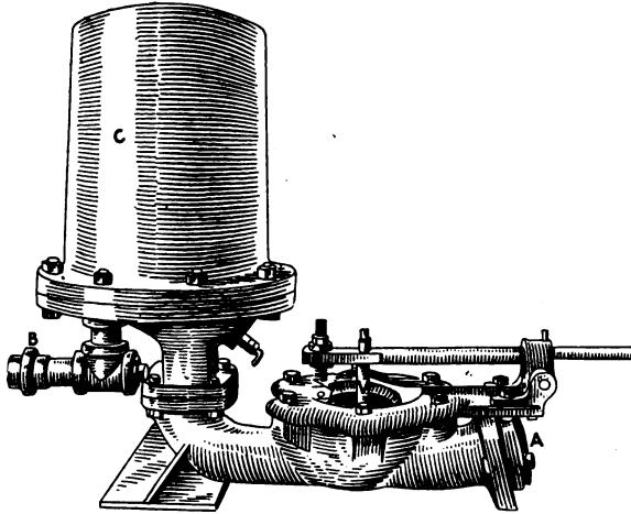
FIG. 215.—Hydraulic ram.
