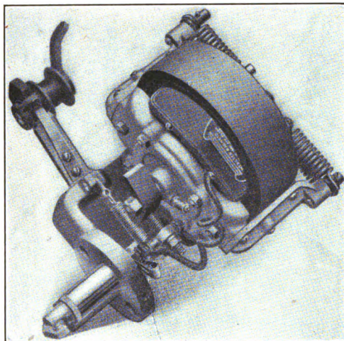
FIG. 100.—Oscillating magneto.
