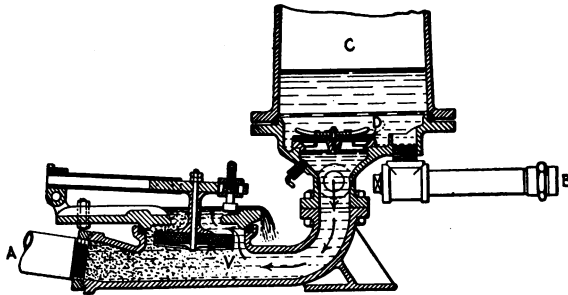
FIG. 214.—Hydraulic ram.
