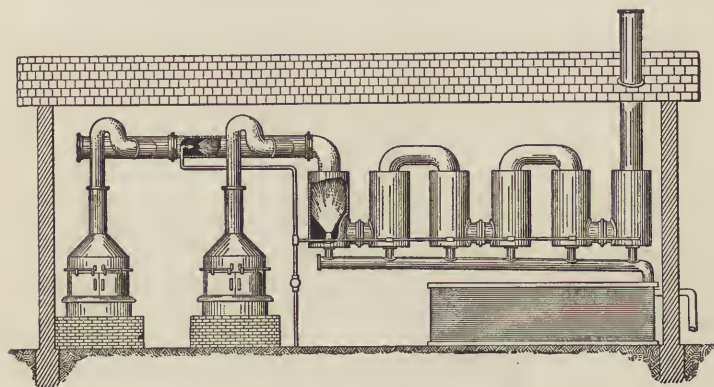
FIG. 20.—Condenser.
