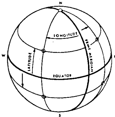
Figure 267 Parallels of Latitude and Meridians of Longitude
