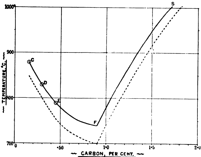
FIG. 54.—Equilibrium diagram.
