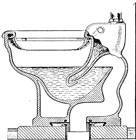
Fig. 25.—Siphon jet closet, "West Point" model (J. L. Mott Co.).
