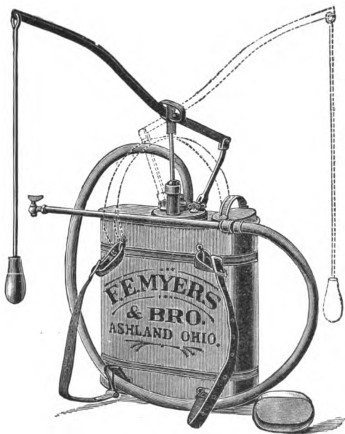
Fig. 27.—“Knapsack” spray pump for oiling standing water (F. E. Myers & Bro.).
