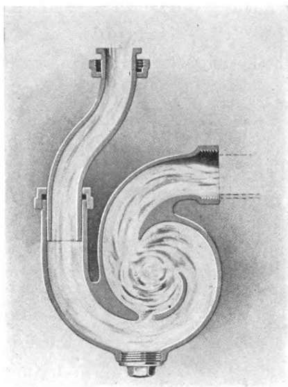
Fig. 26.—Non-siphoning trap vent, "Sanito" model (J. L. Mott Co.).
