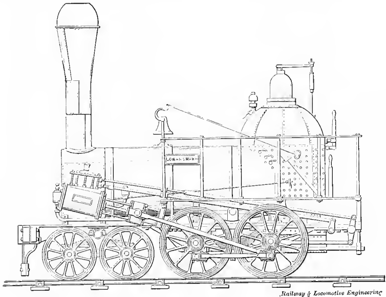
Fig. 74. Gowan & Marx
