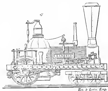
Fig. 109. "Batavia"
