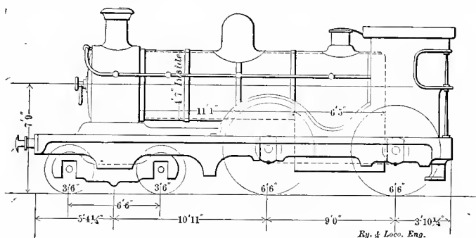
Fig. 27. McIntosh's Dunalistair Class
