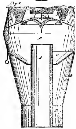
S. Sweet—Pat. Oct 25, 1853
