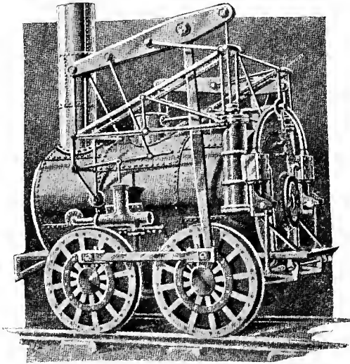
Fig. 28. Stourbridge Lion
