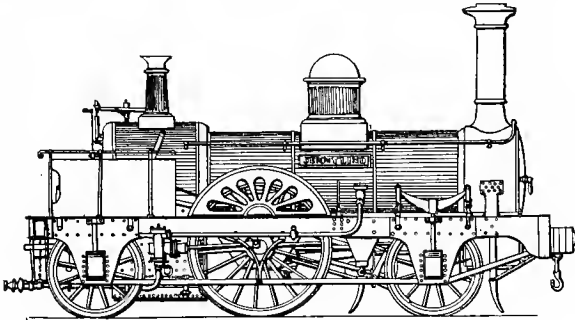
Fig. 18. Joy's Jenny Lind
