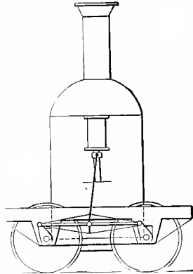
Fig. 37. York
