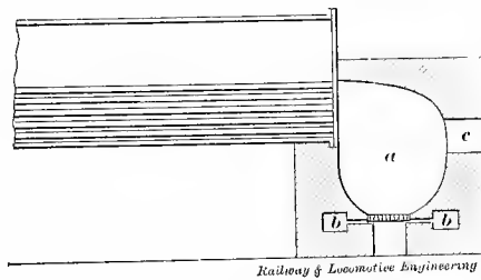
Seguin's Multitubular Boiler, 1827
