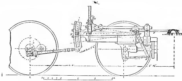
Fig. 226. Mason's Walschaert Motion
