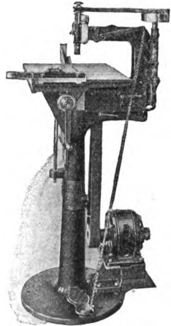
FIG. 119.—Miller Saw-Trimmer.
