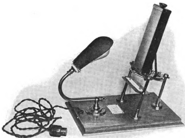
FIG. 352.—Chromo radiometer. (H. W. Cox & Co., Ltd.)
