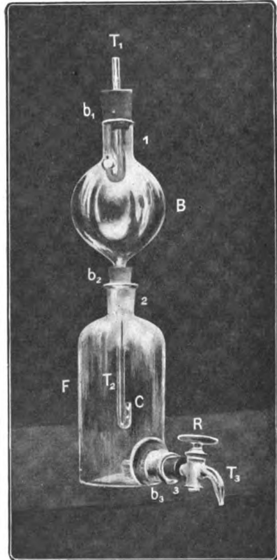
FIG. 388.—Radiogene. (Siemens.)
