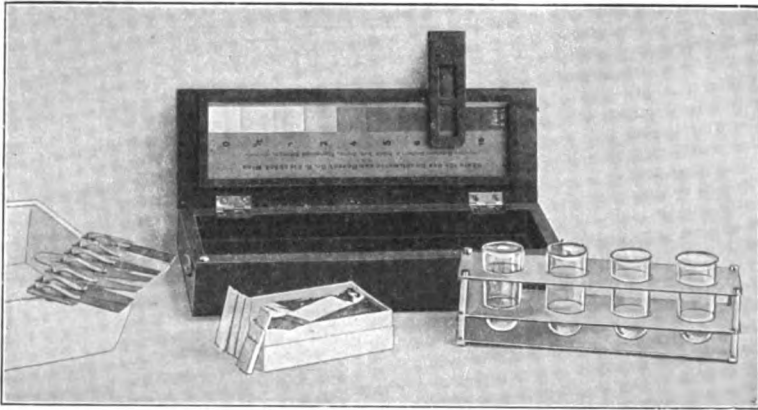
FIG. 341.—Complete Kienböck quantimeter. (Schall.)
