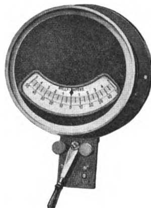
FIG. 324.—Milliamperemeter. (Siemens.)
