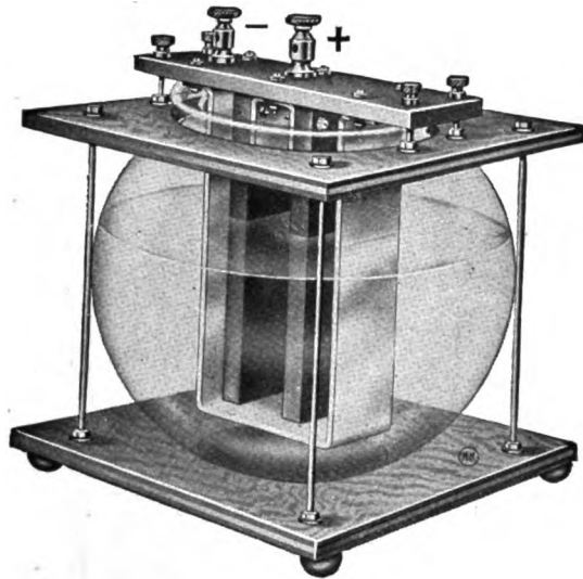
Fig. 27. One-cell rectifier.
