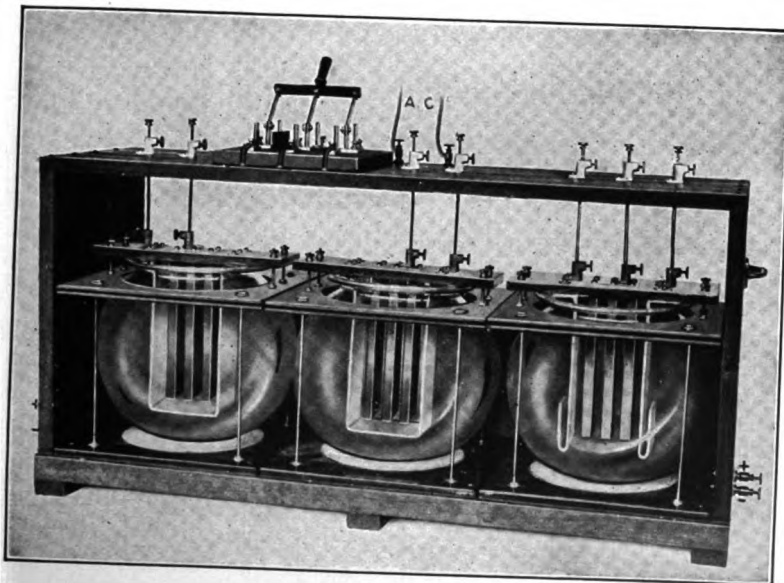
Fig. 28. Three-cell rectifier.
