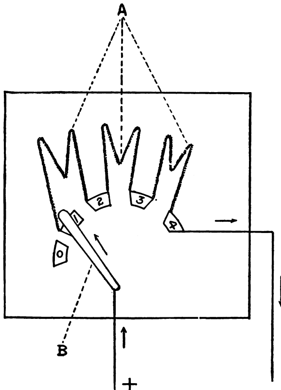
Fig. 30. Diagram of rheostat.
