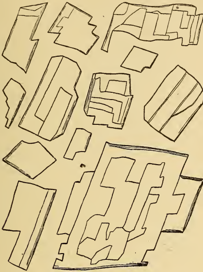
FIG. 42.—CHOLESTERIN CRYSTALS ( \times 400 ).
