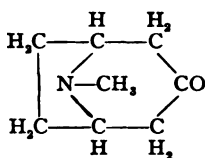
Tropinone (Tropanone)
