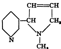
Nicoteline
