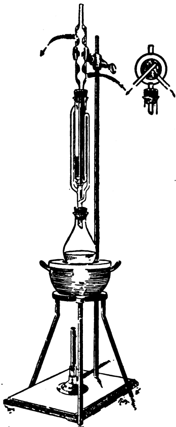
FIG. 113.—SOXHLET APPARATUS.
