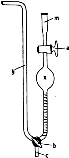
FIG. 103.—FRIDERICIA APPARATUS.
