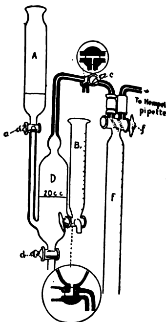
FIG. 35.—SECTION OF VAN SLYKE APPARATUS.
