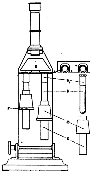
FIG. 94.—BLOOR'S NEPHELOMETER.
