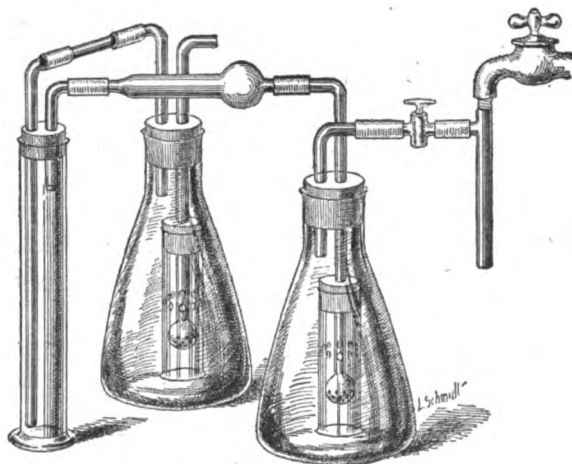
FIG. 167.—FOLIN AMMONIA APPARATUS.
