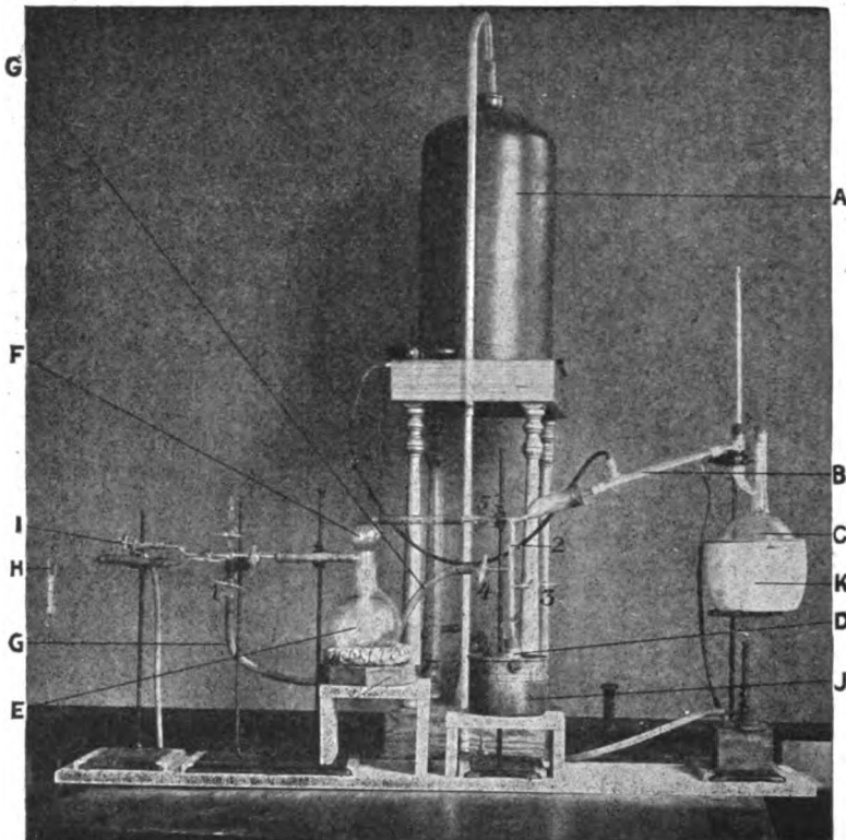
FIG. 24.—FISCHER APPARATUS.
