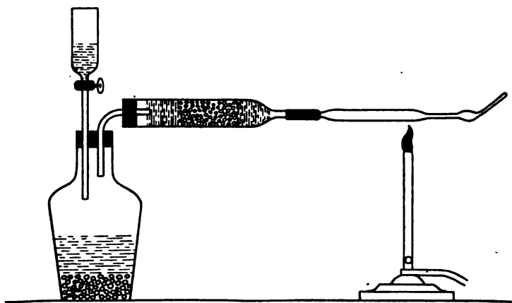
FIG. 137.—MARSH APPARATUS.
