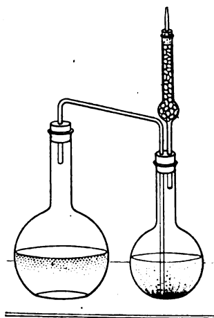
FIG. 3.—FERMENTATION APPARATUS.
