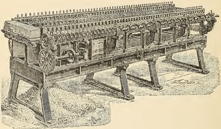
FIG. 4.—The Favier Ramie Machine.
