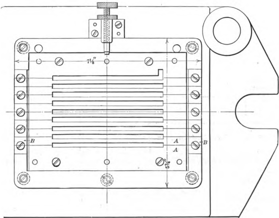
PLAN OF DIE FIG. 115
