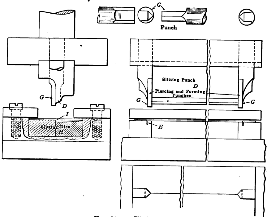
FIG. 361. — Slitting dies
