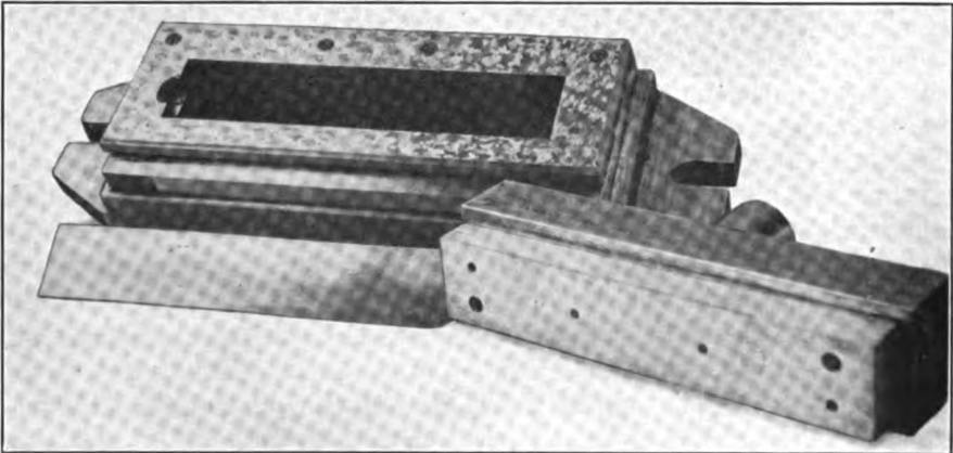
FIG. 391. — The blanking die
