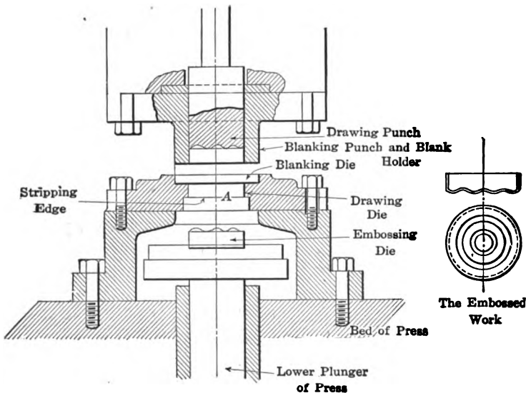
FIG. 25. — Embossing dies
