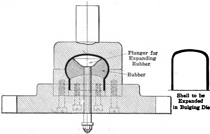
FIG. 19. — Bulging dies
