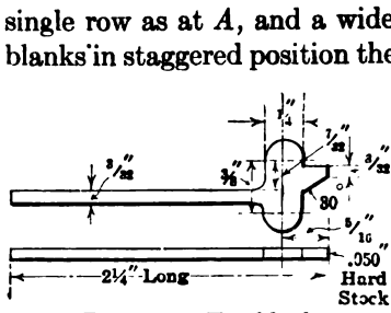
FIG. 41. — The blank
