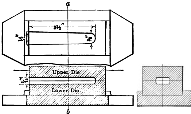
FIG. 24. — Swaging dies
