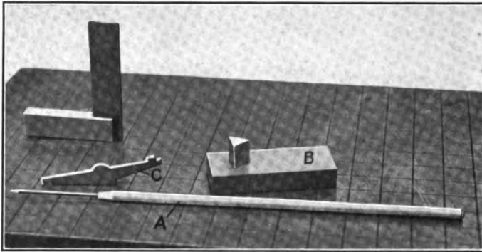
FIG. 550. — Templet tools
