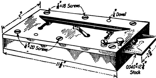
FIG. 369. — The blanking die
