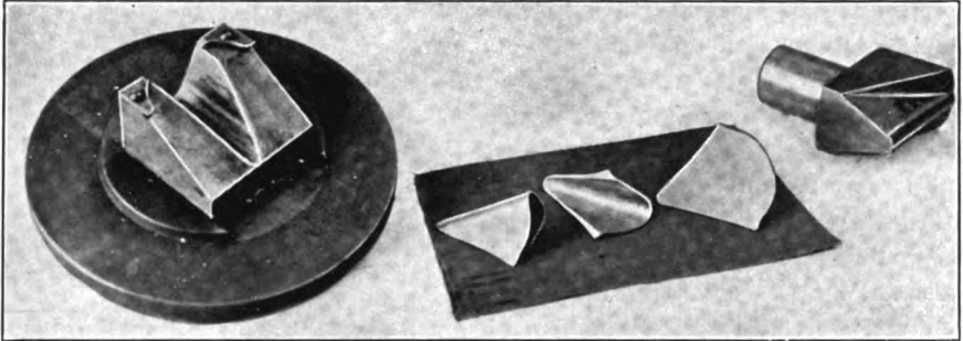
FIG. 20. — Simple bending die
