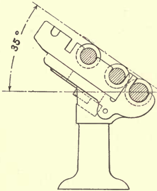
35° ROLL STAND
