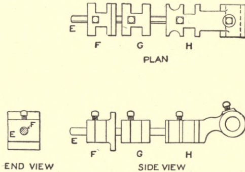
Fig. 180. Cap Bar.
