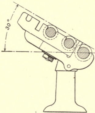
30° ROLL STAND
