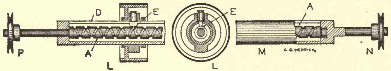
Fig. 90. Traverse Grinder.
