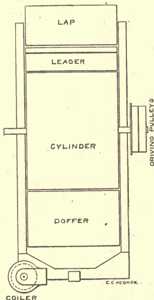
Fig. 61. Plan of R. H. Card.
