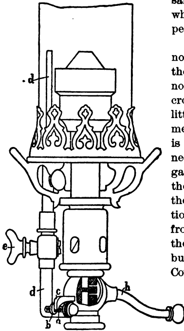
FIG. 37.—BURNER OF FISCHER & CO.
