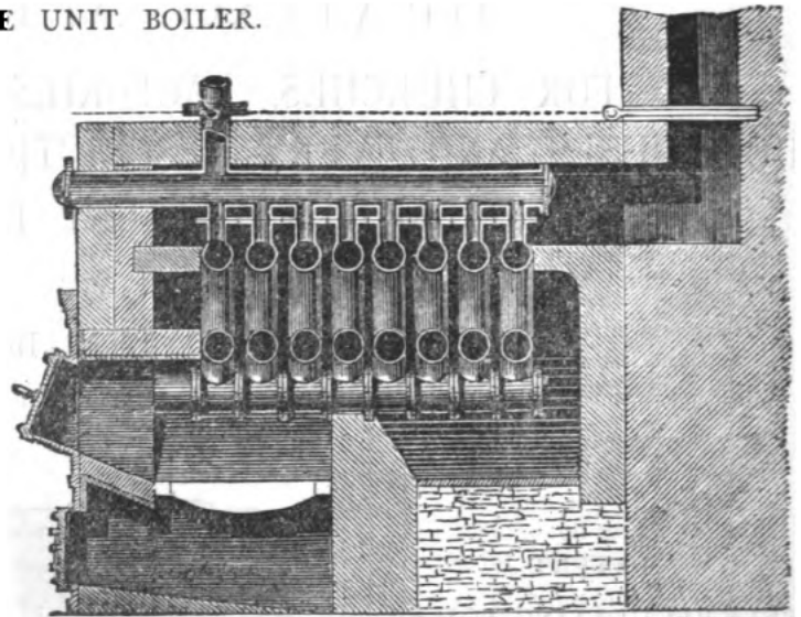
LONGITUDINAL SECTION.
