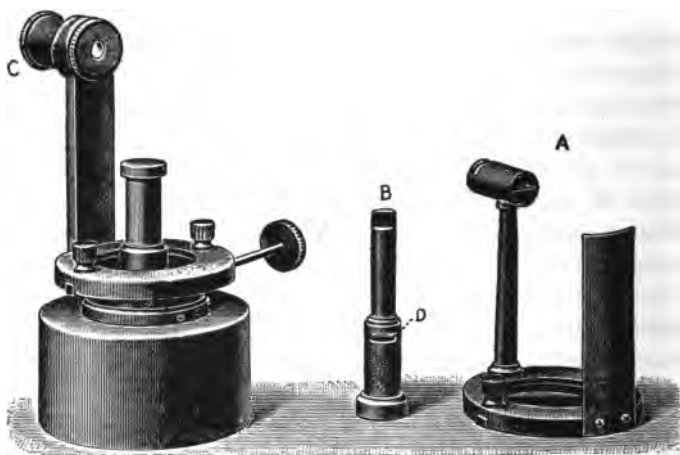
FIG. 27.—Hefner lamp.
