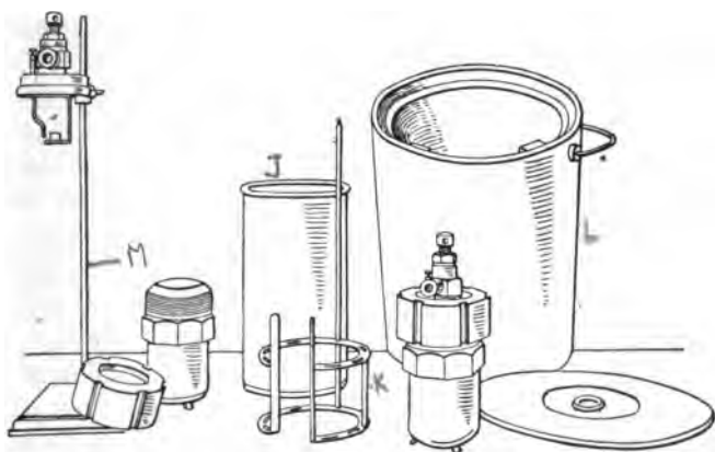
FIG. 56.—Bomb calorimeter.
