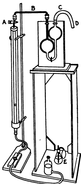
FIG. 5.—Gas burette and pipette.
