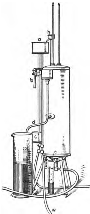
FIG. 22a.—Gas calorimeter.
