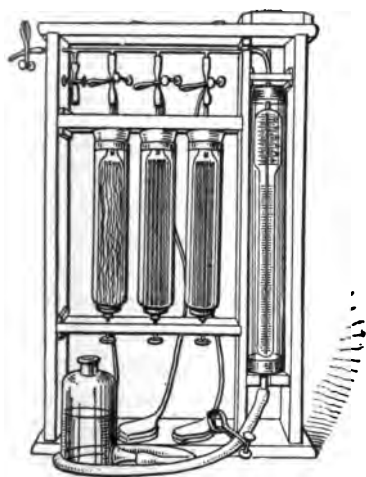
Fig. 16.—Orsat apparatus. Allen-Moyer modification.
