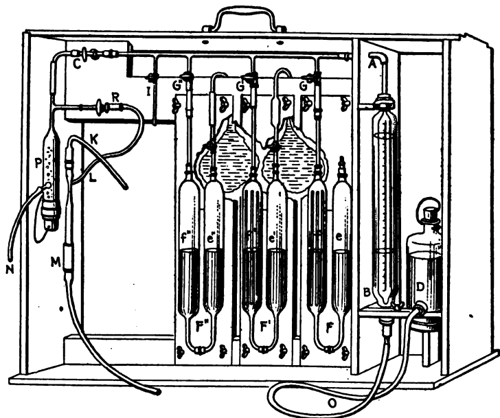
FIG. 15.—Orsat apparatus. Original form.
