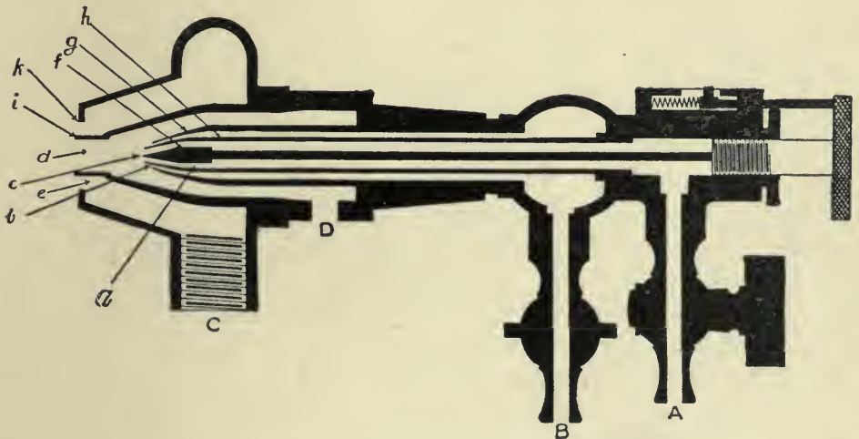
Fig. 65. HÖVELER ATOMIZER.
