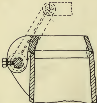
Fig. 31. MACALLAN VARIABLE BLAST CAP.
