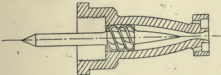
Fig. 22a. KÖRTING ATOMIZER.
