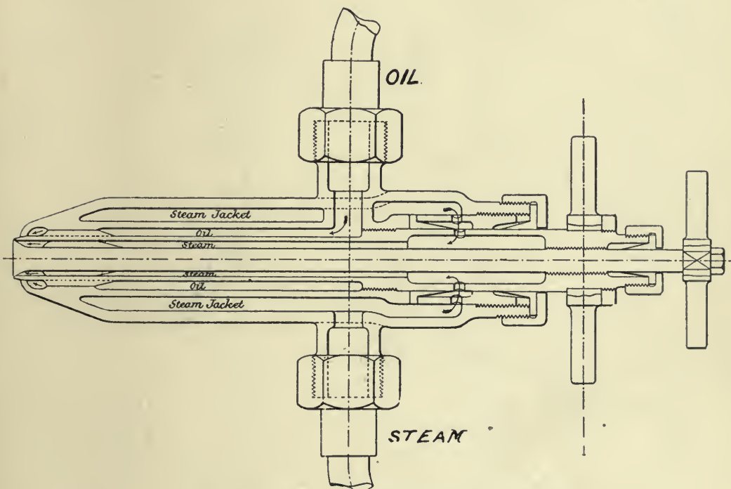
Fig. 66. ATOMIZER. RUSDEN-EELES.
