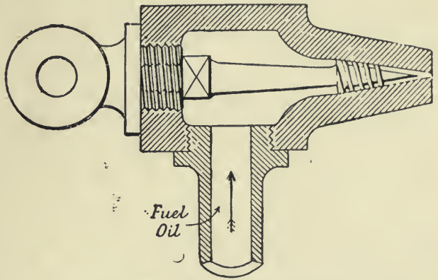
Fig. 22. KÖRTING ATOMIZER.
