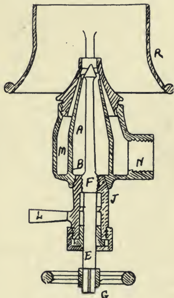
Fig. 79. D'ALLEST ATOMIZER.
