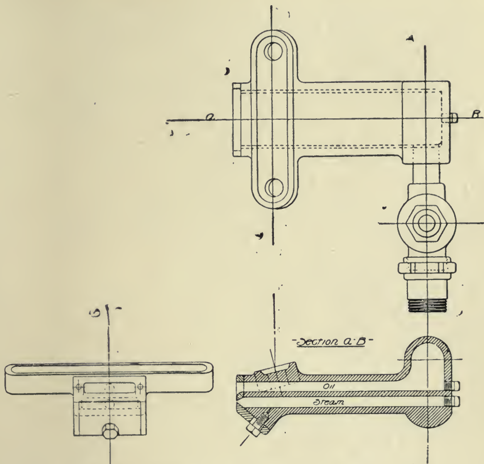
Fig. 34. ATOMIZER. BALDWIN LOCOMOTIVE CO.
