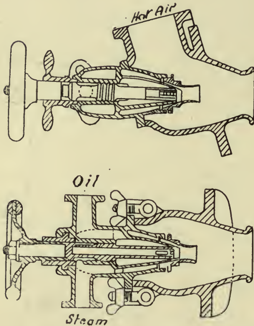
Fig. 80. D'ALLEST DOUBLE ATOMIZER.
