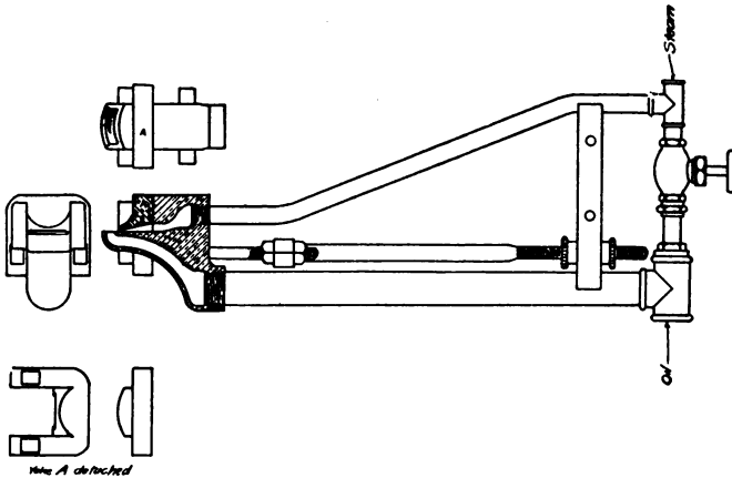
Fig. 22. N. N. Best Burner.
