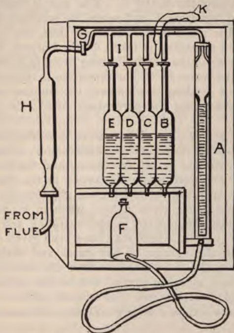
Fig. 107. Orsat Apparatus.
