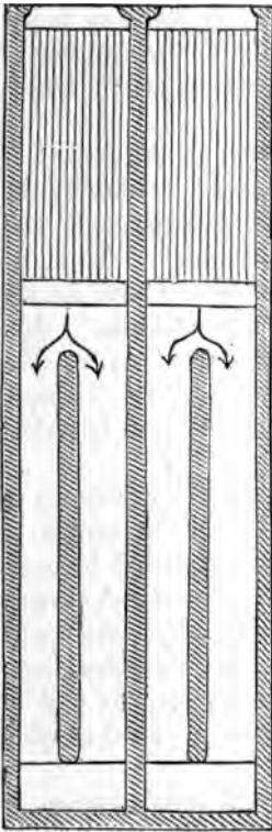
Fig. 95.—Split Draught.
