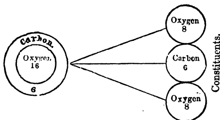
Fig. 5.—Carbonic Acid.
