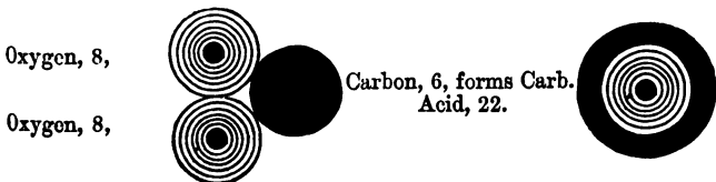
Fig. 6.—Carbonic Acid.
