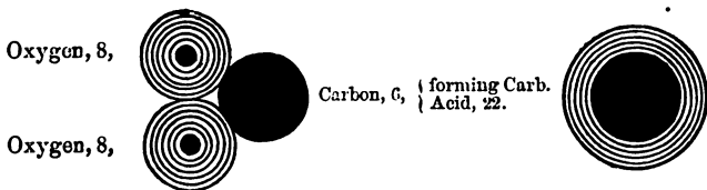
Fig. 8.—Carbonic Acid.
