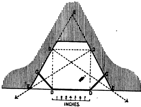
FIG. 29.—"Economiser" Fireplace.
