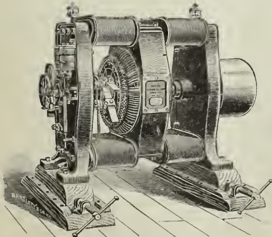
Wood Dynamo.
