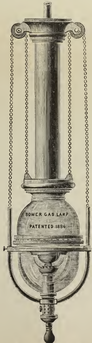
Fig. 3.—Exterior View.
