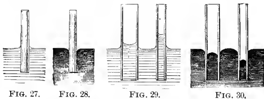
FIG. 27. FIG. 28. FIG. 29. FIG. 30. CAPILLARY PHENOMENA. (Gannot.)
