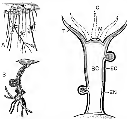
FIG. 57.—HYDROZOA. (Jeffrey-Bell.)
