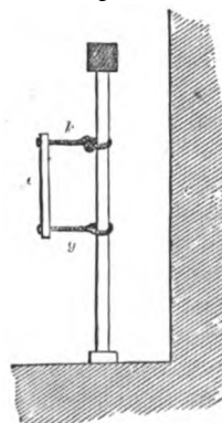
A BAIKIE.
