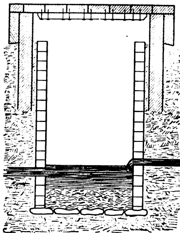
Fig. 140. Silt basin.
