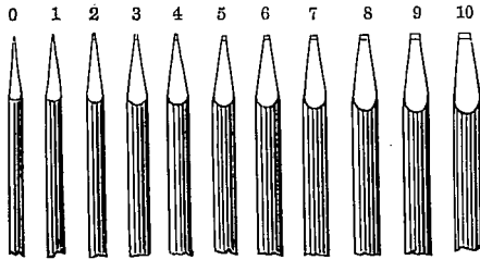
Fig. 20. TINT-TOOLS.
