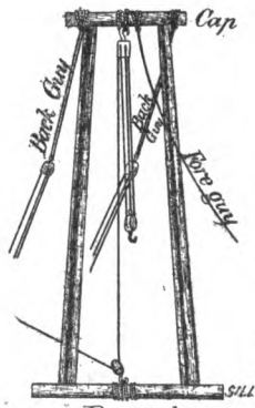
Derrick
