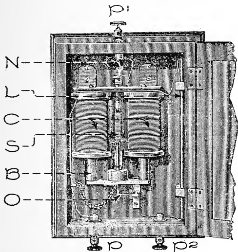
CONTROLLER FOR ARC DYNAMO.
