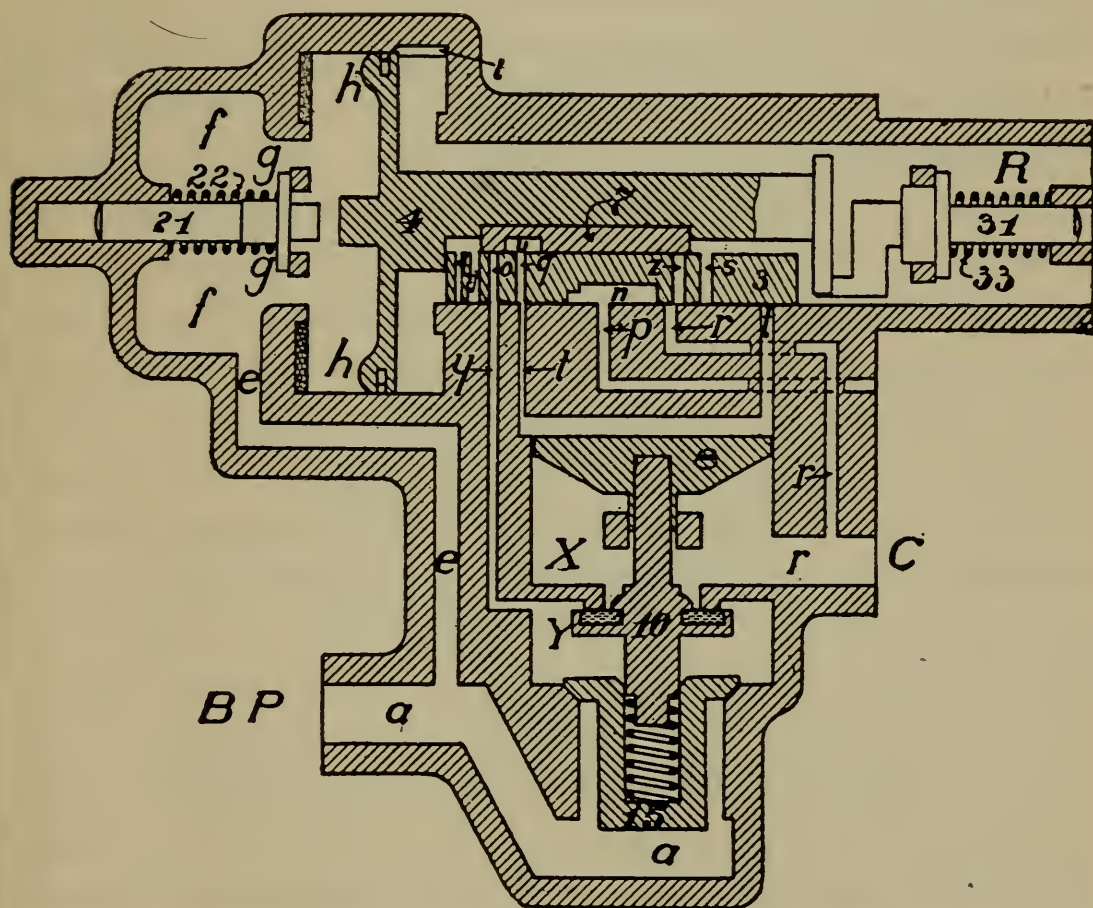
FIG. 329. LAP POSITION
