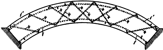
FIG. 187.—Melber patent.
