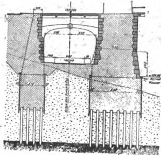
Fig. 18. Schnitt Z-Z durch den Träger.
