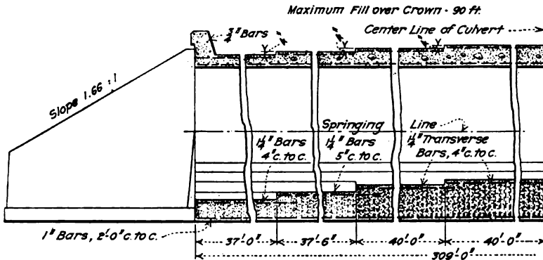
FIG. 330.—Double-barrel culvert, D. L. & W. R. R.
