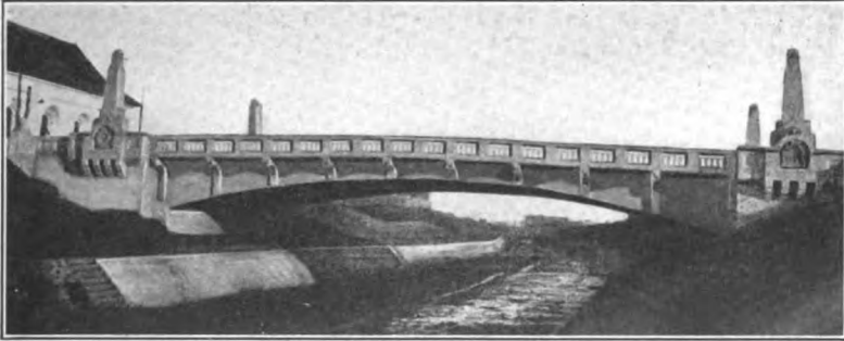
From "Handbuch für Eisenbetonbau." FIG. 526.—Mühlplatz bridge over Béja Canal in Temesvár, Hungary.
