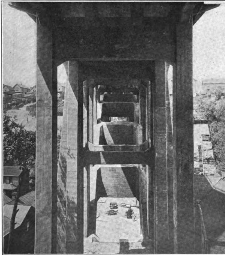
FIG. 228. —Monessen viaduct, Monessen, Pa.
