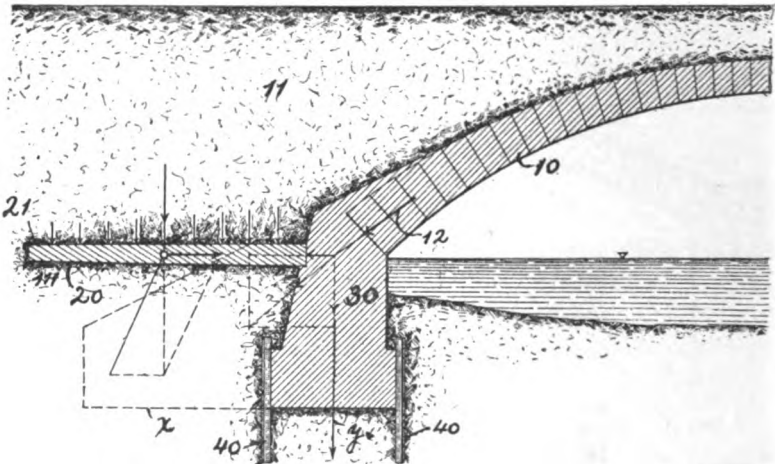
FIG. 193.—Moller patent.
