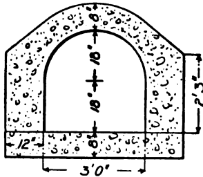
Fig. 171.—Small Culverts, Pennsylvania R. R.
