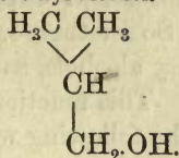
Isobutyl alcohol.
