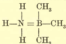
Ammonio-boron Methide.
