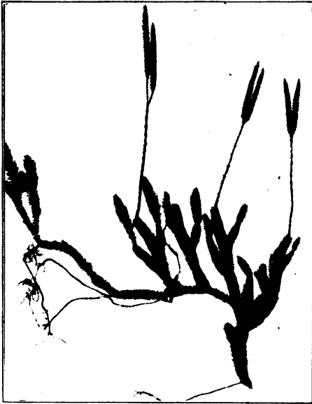
FIG. 272.— Lycopodium clavatum .
