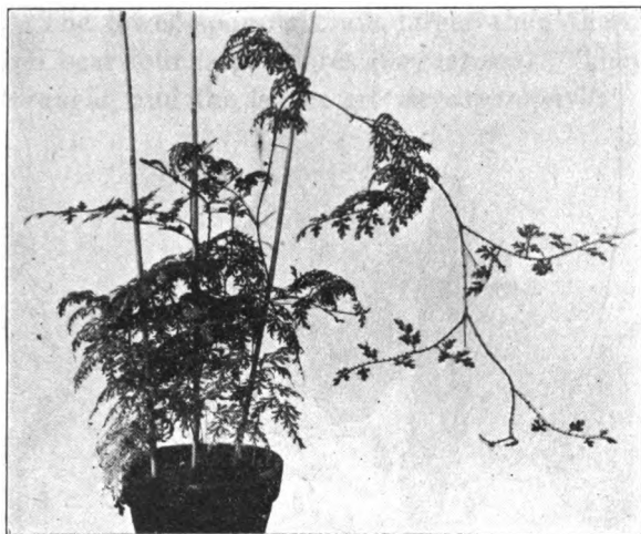
FIG. 277.— Selaginella Wildenovii .
