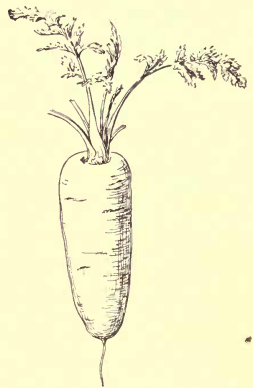
FIG. 52. — Carrot.
