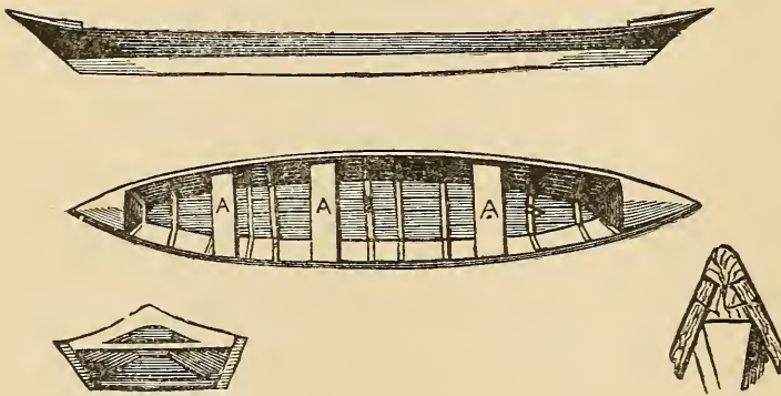
Fig. 10.—Canadian Batteau.
