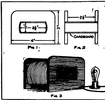
Watch Demagnetizer
