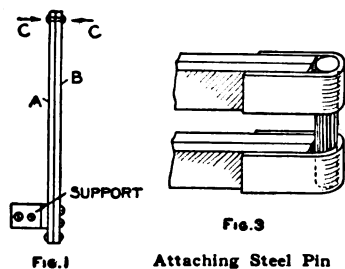
Simple Thermostat
