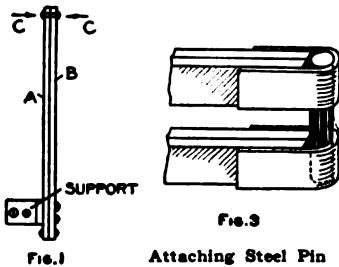
Simple Thermostat
