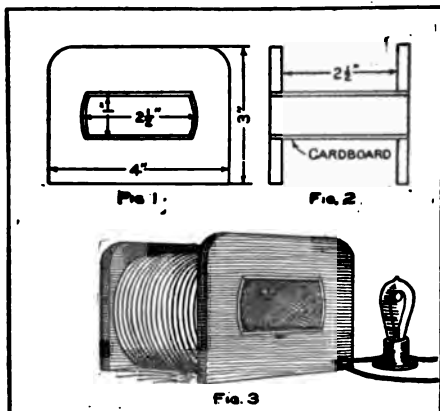
Watch Demagnetizer
