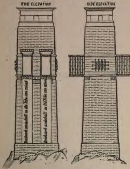
FIG. 98.—Britannia Tower.
