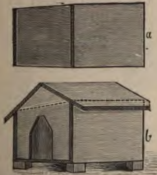
FIG. 62.—Dog Kennel.
