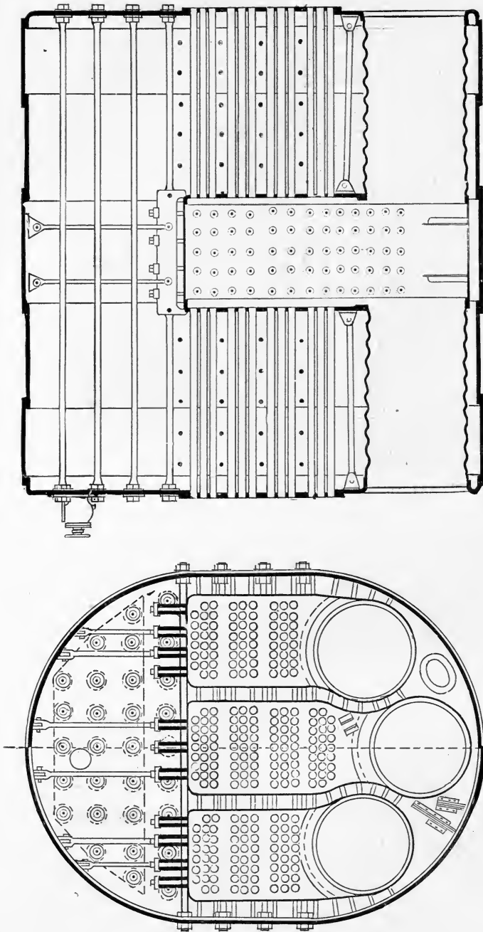
BOILERS FOR S. S. "MEXICAN."
