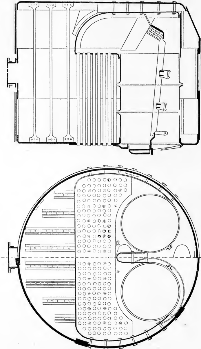
BOILER OF H. M. S. "ROVER."
