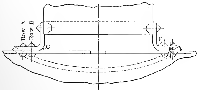
FIG. 42.—DOME COLLAR.
