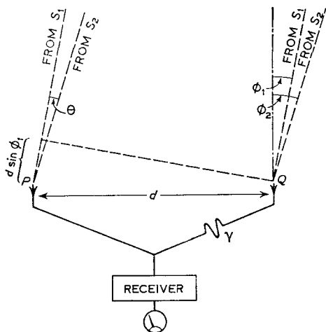
Fig. 25. The Michelson stellar interferometer
