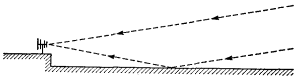
Fig. 26. The sea interferometer
