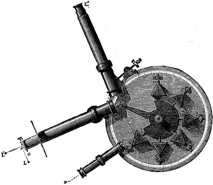
FIG. 143.—SPECTROSCOPE
