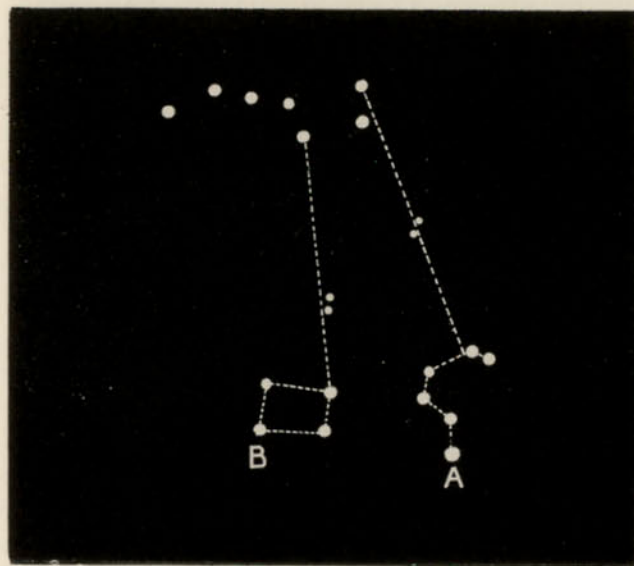
A, Regulus. B, Denebola.
