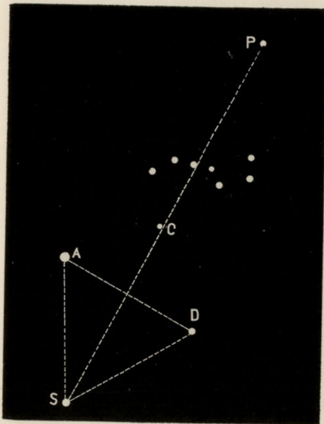
P, Polaris. C, Cor Caroli. A, Arcturus. D, Denebola. S, Spica.
