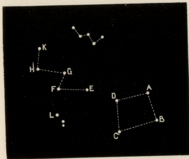
A, Beta Pegasi. B, Alpha Pegasi. C, Gamma Pegasi. D, Alpha Andromedae. E, Beta Andromedae. F, Beta Trianguli. G, Gamma Andromedae. H, Beta Persei. K, Alpha Persei. L, Alpha Arietis.
