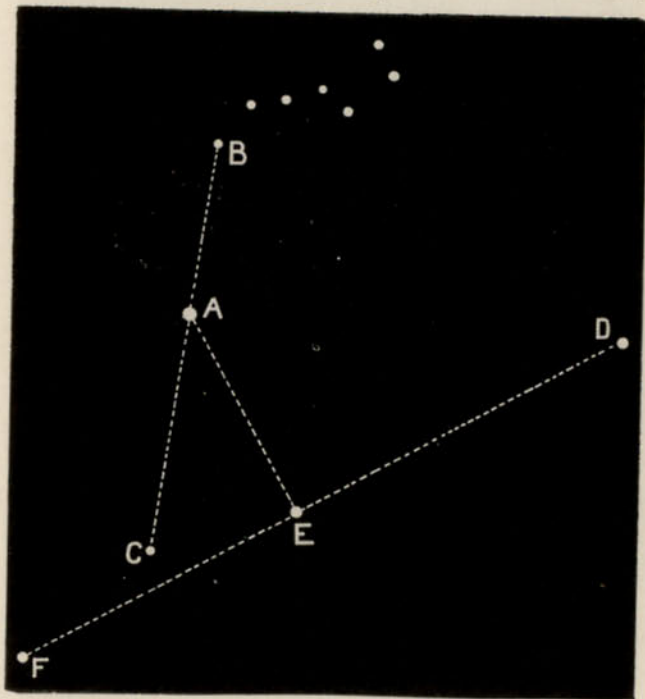
A, Arcturus. B, Alkaid. C, Alpha Libræ. D, Regulus. E, Spica. F, Antares.
