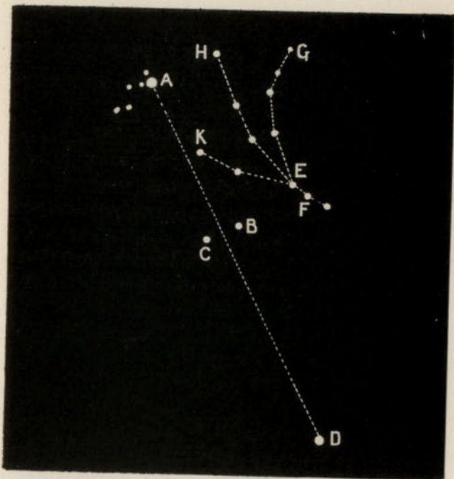
A, Vega. B, Ras al Gethi. C, Ras al Hague. D, Antares. E, Beta Herculis. F, Gamma Herculis. G, Tau Herculis. H, Iota Herculis. K, Mu Herculis.
