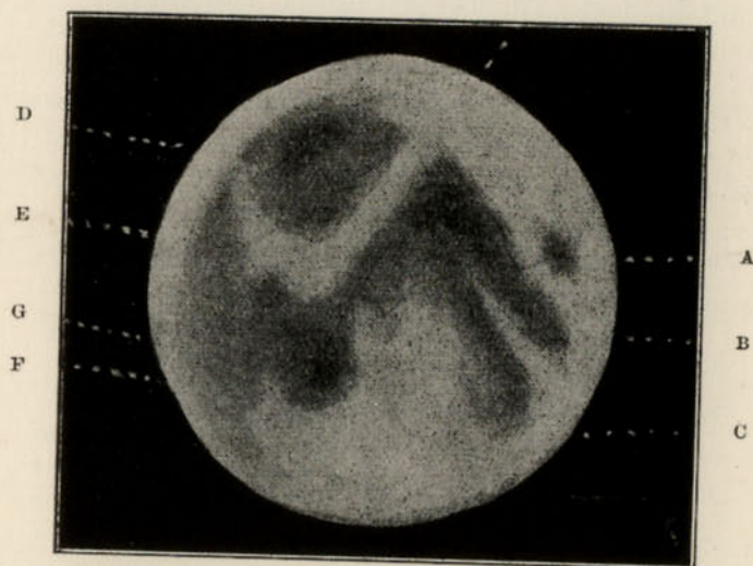
A, Mare Crisium. B, Mare Fœcunditatis. C, Maria Nectaris et Tranquillitatis. D, Mare Imbrium. E, Oceanus Procellarum. F, Mare Humorum. G, Mare Nubium. H, Apennines and Copernicus.
