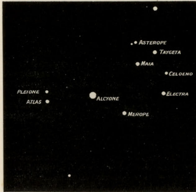
FIG. 21.—The Pleiades.
