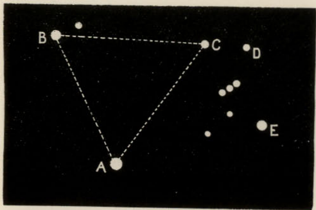
A, Sirius. B, Procyon. C, Betelgeuse. D, Bellatrix. E, Rigel.
