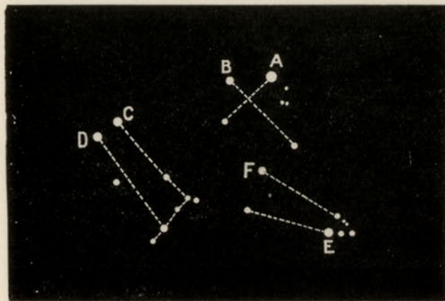
A, Capella. B, Menkalinan. C, Castor. D, Pollux. E, Aldebaran. F, Almath.
