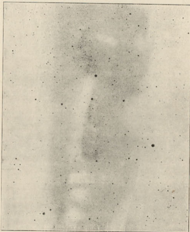
FIG. 38.—The Milky Way in Cygnus. From Mr. C. Easton's "La Voie Lactée."
