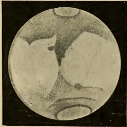
FIG. 41.—Telescopic aspect of the planet Mars (Feb., 1901).
