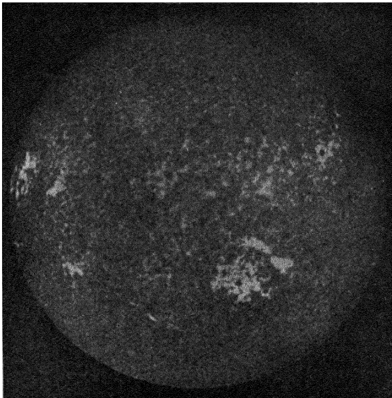
· Diag. LX.—Calcium Flocculi.
