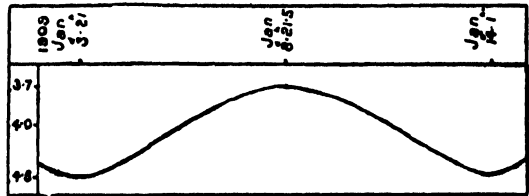
Diag. XCIII. Light changes of ζ Geminorum.
