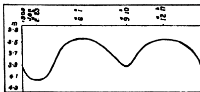
Diag. XCI. Light changes of \beta Lyrae.
