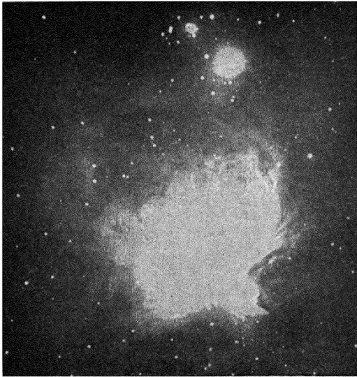
Diag. LXXX.—Orion Nebula.
